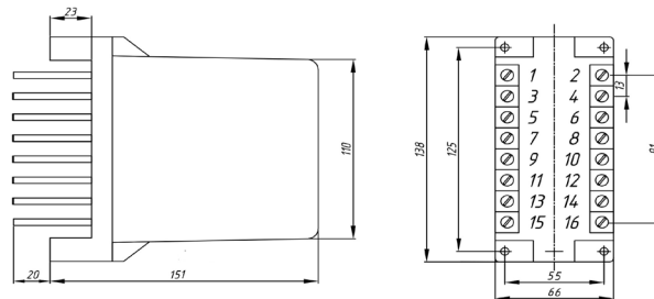
б) заднее присоединение шпилькой
