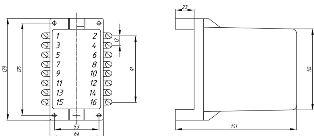
а) переднее присоединение винтовыми зажимами
