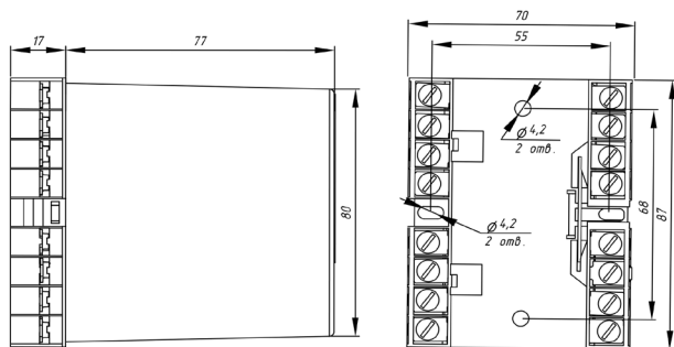
б) заднее присоединение винтовыми зажимами
