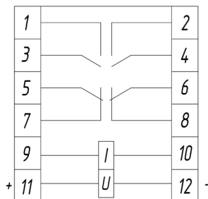
Рисунок 6. Схема подключения РПм-16-4 на базе основания ОР002 и ОР003.
